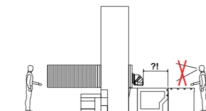
COMPETITOR SOLUTION 2 Lateral moving column machine - Macchina aggraffata - Maschine mit rückseitiger Zusatzführung - Machine à montant mobile latéral
