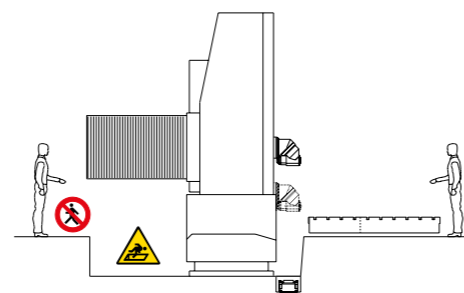
COMPETITOR SOLUTION 1 Traditional foundation with pit - Fondazione tradizionale a fossa - Traditionelle Fundamentgrube - Fondation traditionnelle avec fosse
