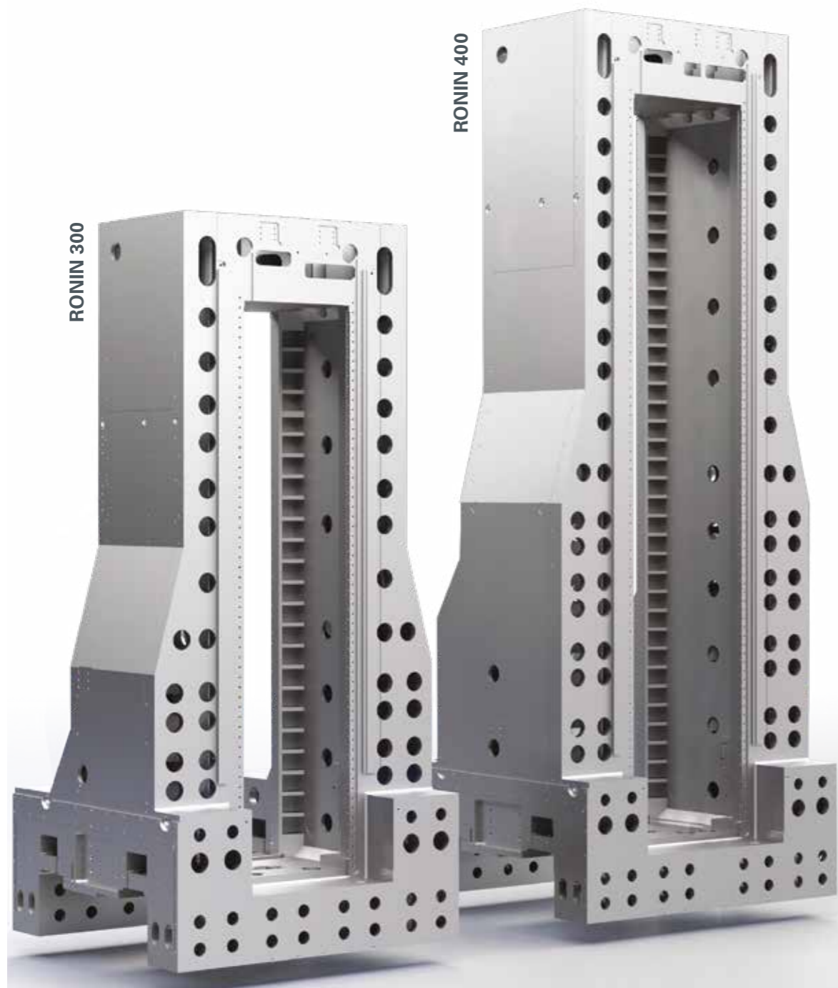
The column of Ronin 400 with V=4000 compared with the column of Ronin 300 with V=3000 Il montante della Ronin 400 con V=4000 a confronto con quello Ronin 300 V=3000 Der Ständer Ronin 400 mit V=4000 gegenüber dem Ständer Ronin 300 mit V=3000 Le montante de la Ronin 400 avec V=4000 par rapport au montante de la Ronin 300 avec V=3000
